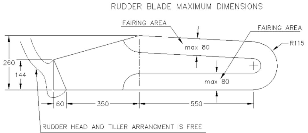
E.4.4.1. RUDDER DIAGRAM
